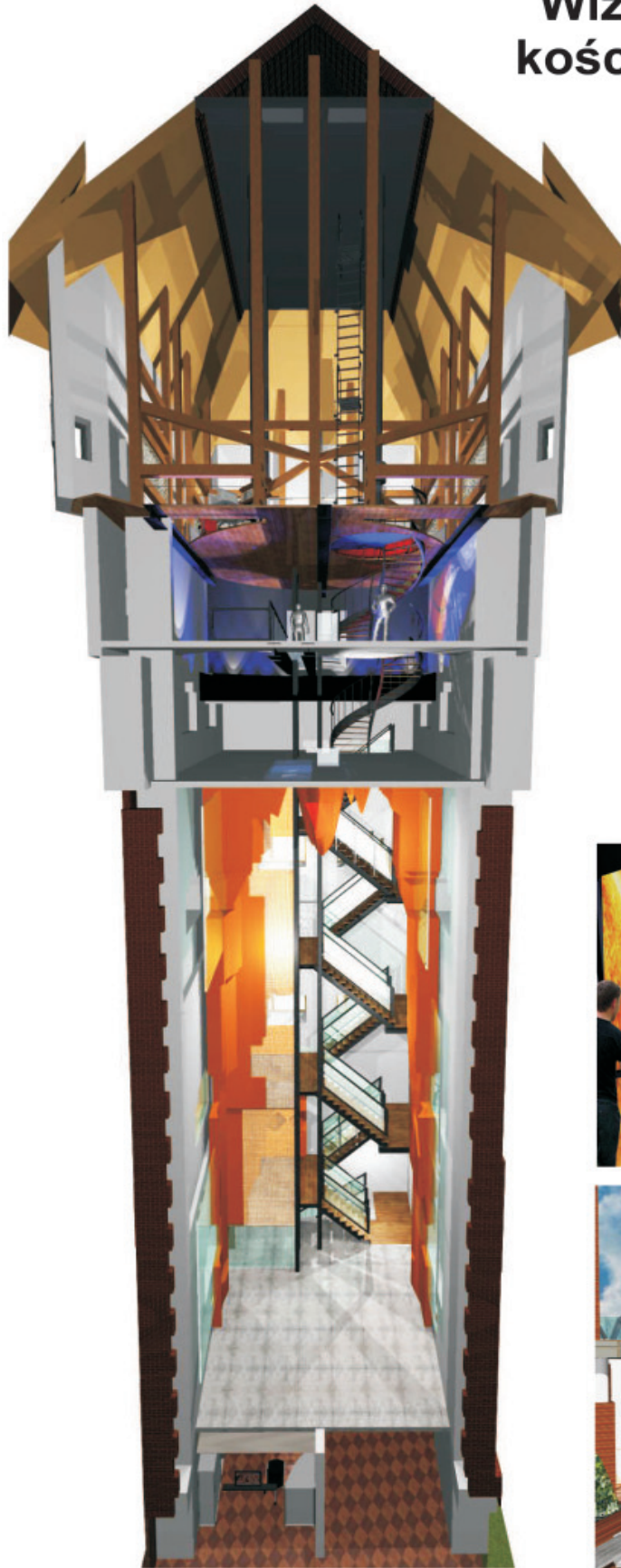
Przekrój Wieży Ciśnień
